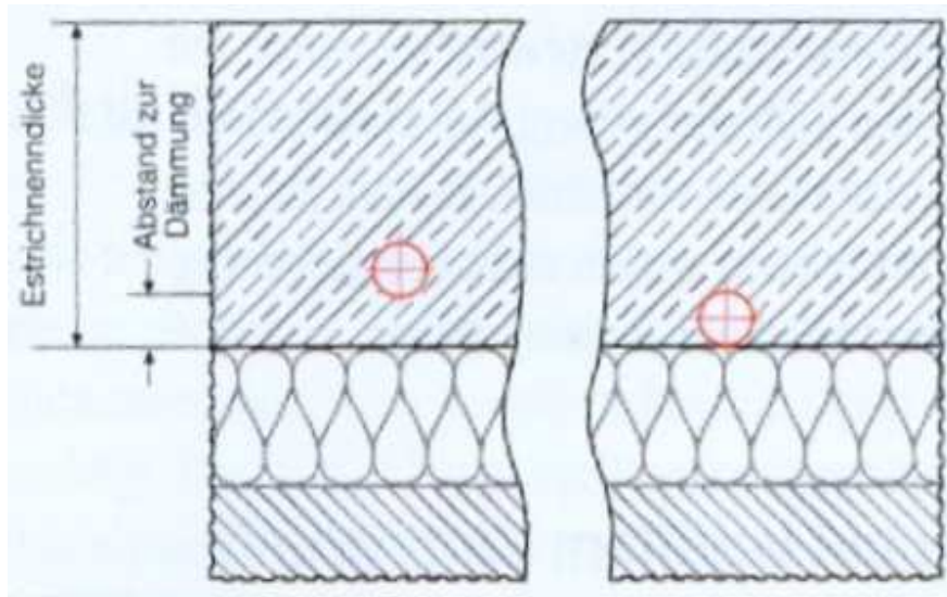
Bild 1: Mögliche Heizrohranordnungen bei Heizestrich Bauart A ergeben unterschiedliche Überdeckungshöhen (Dicke des Estrichs über Oberkante Heizrohr).
