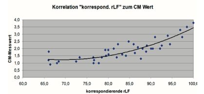
Grafik 1: Labormessungen an Zementestrichen, Mischungsverhältnis 1:4 – 1:6, w/z-Wert 0,4 bis 0,7
