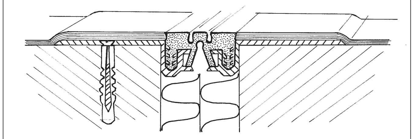
Bewegungsfugensystem von Migua zum nachträglichen Einbau
