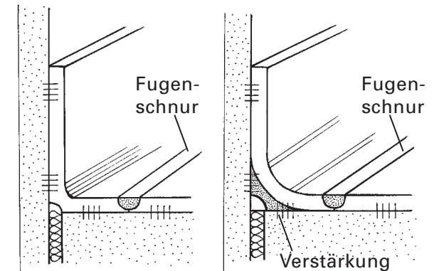
Sockelstreifen gefräst
